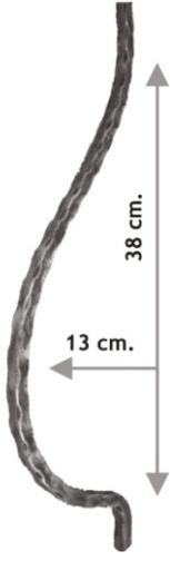
2541 500mm-710gr Ø12x12
