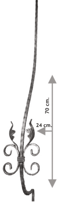
2503 1250mm-2025gr 1500mm-2307gr Ø12x12
