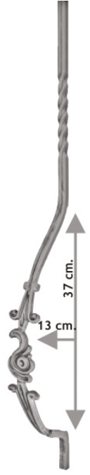
2478 800mm-1090gr 1000mm-1310 Ø12x12
