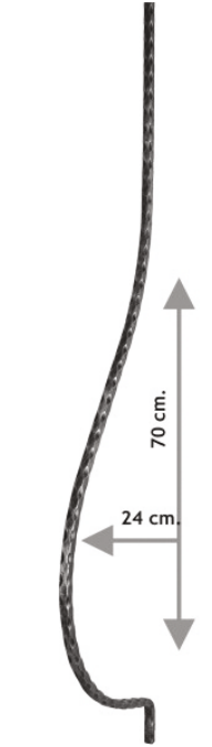
2509 1000mm-1190gr 1250mm-1470gr 1500mm-1750gr Ø12x12
